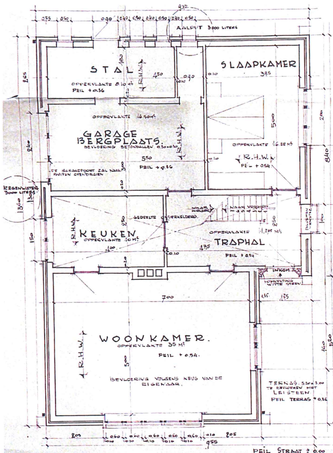
PLAN GELUKVLOERS
