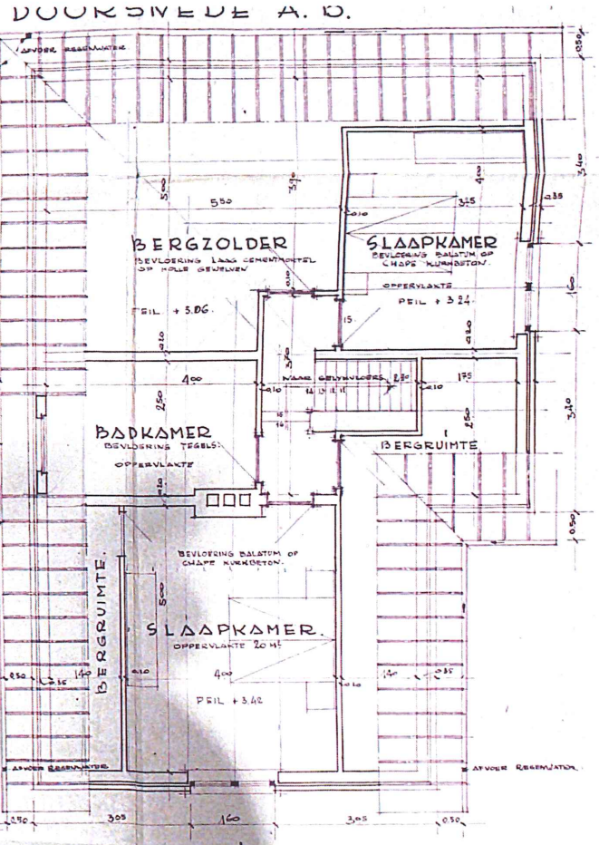
PLAN VERDIEP.
